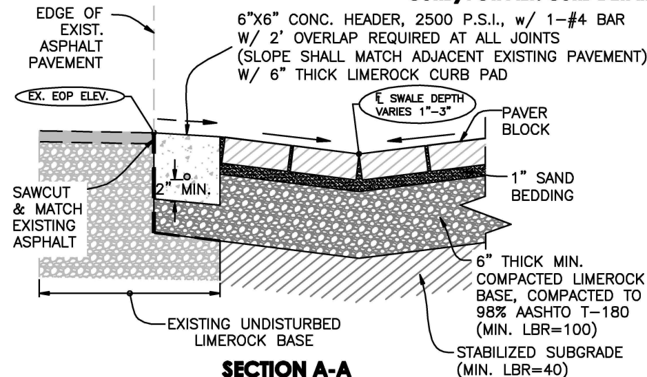
ALTERNATE HEADER CURB DETAIL N.T.S.
