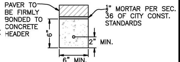
ALTERNATE HEADER CURB DETAIL N.T.S.
